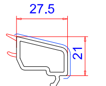
Штапик 27.5мм Арт.-№: 107.143 для с/п 24мм
