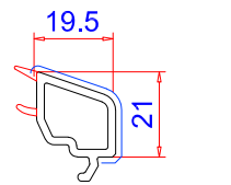
Штапик 19.5мм Арт.-№: 107.215 для с/п 32мм
