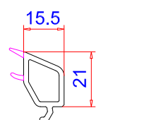
Штапик 15.5мм Арт.-№: 107.217 для с/п 36мм
