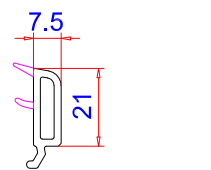
Штапик 7.5мм Арт.-№: 107.228 для с/п 44мм
